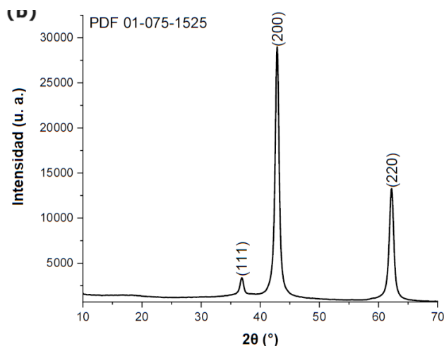
Fig. 1. Espectros IR de la muestra de precalcina a 300 °C y del sólido calcinado a 500 °C (a) y difractograma de rayos X del sólido tratado térmicamente (b).
