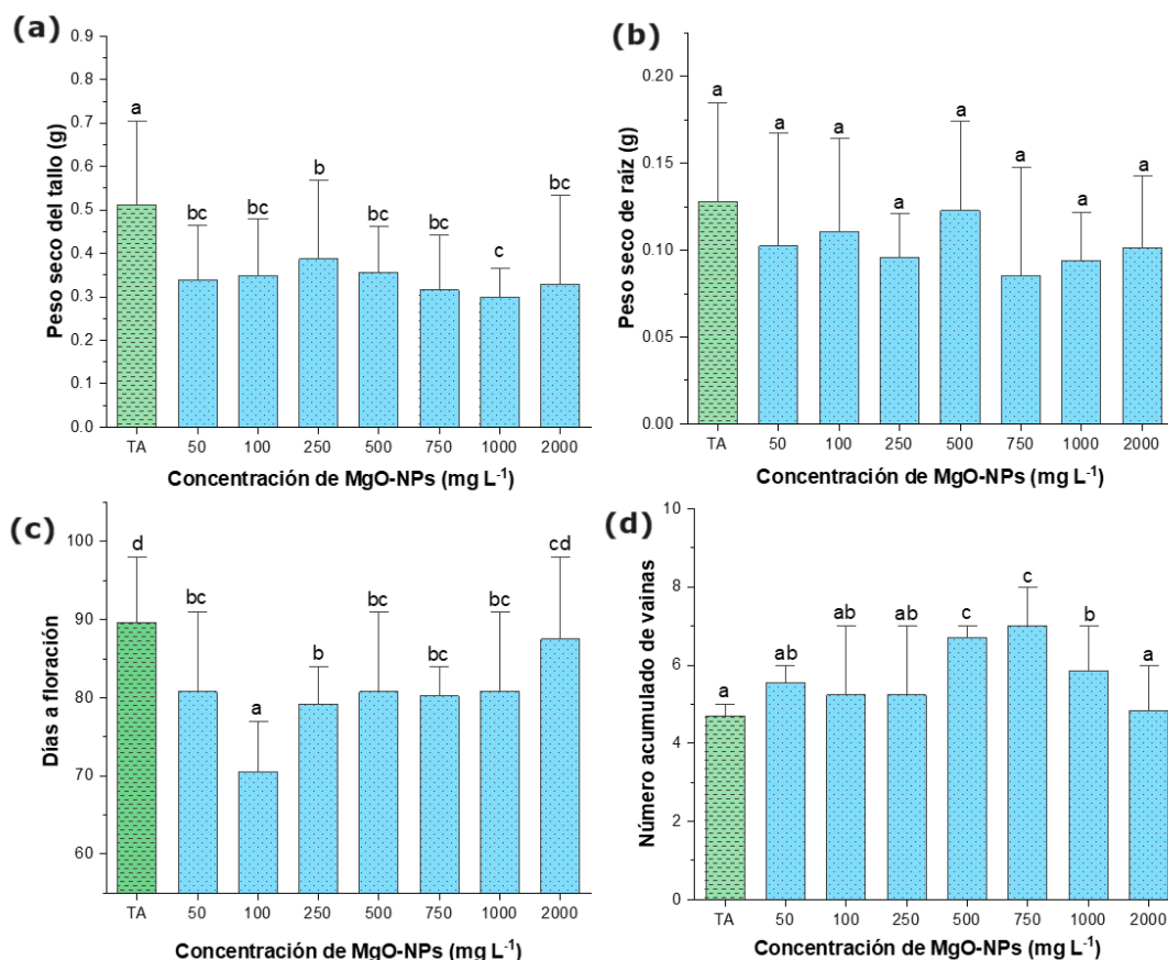
Fig. 3. Masa seca de tallos (a), masa seca de raíces (b), días a floración (c) y número acumulado de vainas por planta (d), estimados en plantas de V. unguiculata obtenidas de semillas tratadas con MgO-NPs en concentraciones de 0 (TA), 50, 100, 250, 500, 750, 1000 y 2000 mg L -1 . [El asterisco (*) indica que el tratamiento es estadísticamente diferente a TA, ns indica que con relación a TA no existe diferencia significativa ( p < 0.05 ) y la línea sobre la barra corresponde a la desviación estándar, n = 10 ].
