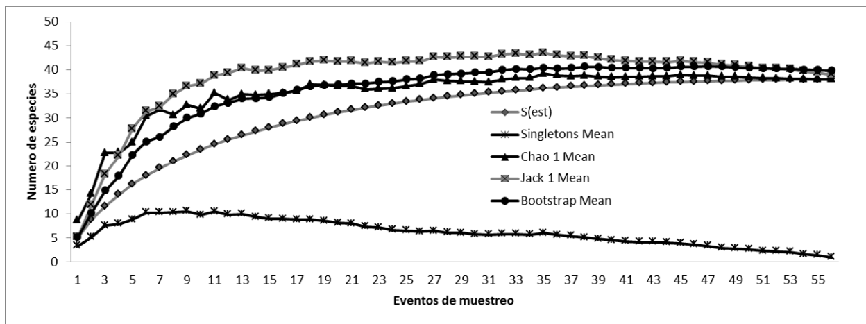
Figura 1. Curva de acumulación de especies de murciélagos y su respectiva representatividad para todos los estados sucesionales.
