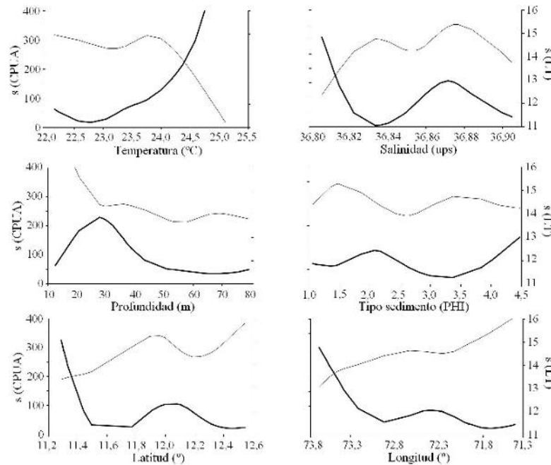
Figura 9. Resultados de la modelación GAM de las relaciones funcionales entre las tallas (cm) (línea delgada), CPUA ( \text{kg}/\text{km}^2 ; línea gruesa) de E. argenteus con los predictores (temperatura, salinidad, profundidad, tipo de sedimento, latitud y longitud).
