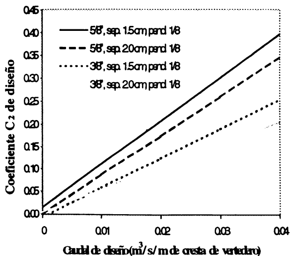
GRÁFICA 9. Coeficiente de contracción C_2 de diseño en función del caudal captado
