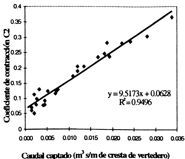
GRÁFICA 8. Coeficiente de contracción C_2 para rejilla de barras \phi 5/8" , separadas 1.5 cm y con una pendiente de 1/8 .
