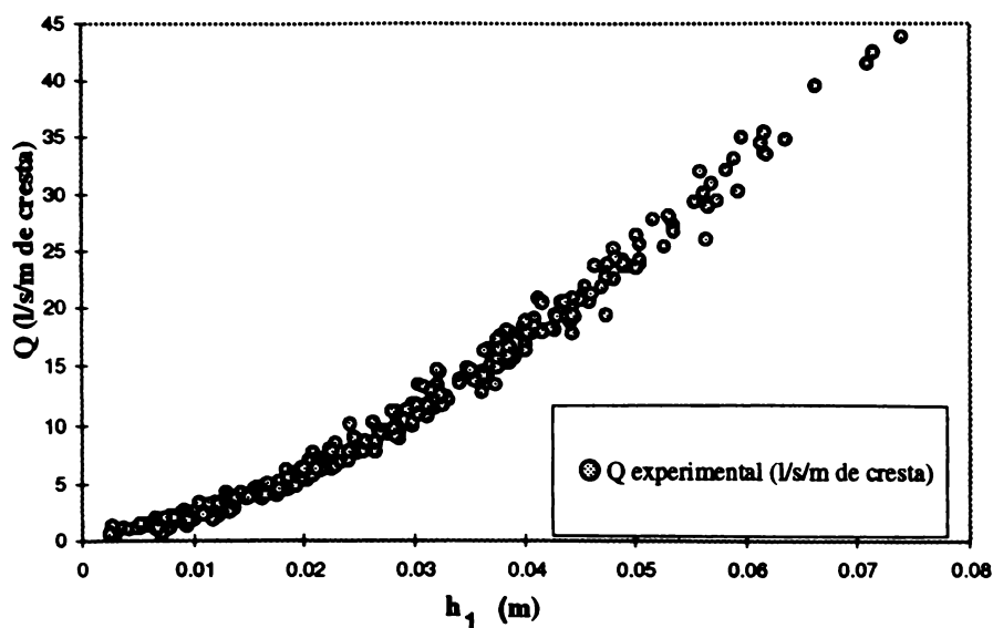
GRÁFICA 3. Valores del caudal aforado por metro lineal de cresta en función de h_1 (m) experimental, para todos los casos.
