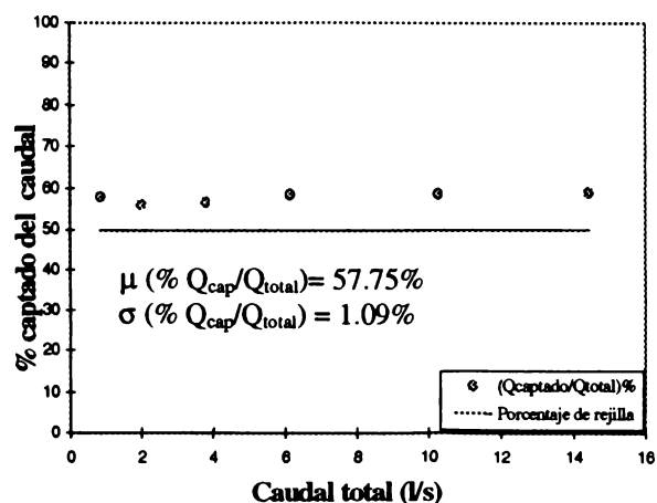
GRÁFICA 5. Porcentaje captado del caudal total, con rejilla de barras \phi 5/8'' separadas 1.5 cm ocupando un 50% del vertedero de rebose, con pendiente 1/6.
