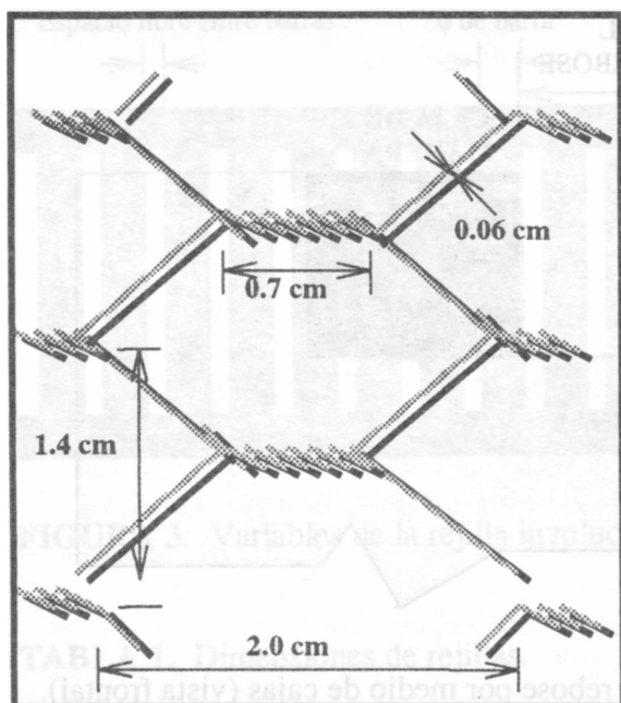
FIGURA 7a). Malla de “pajarito”.
