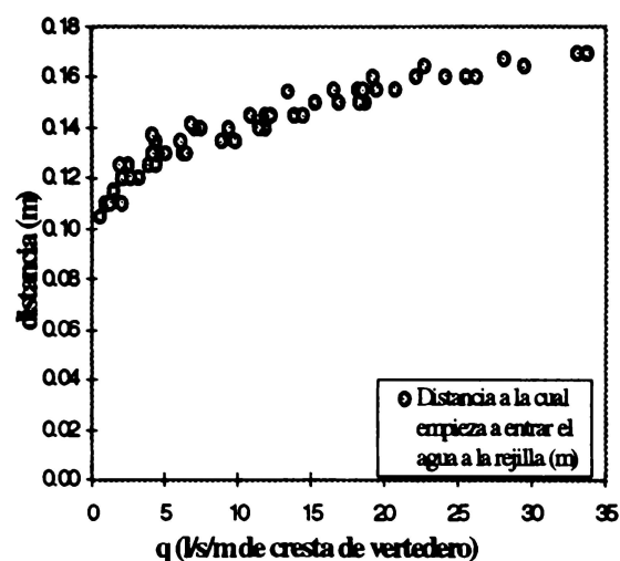
GRÁFICA 6. Distancia B' a la cual entra el agua en la rejilla de barras \phi 5/8'' , separadas 1.5 cm, para una pendiente de vertedero de 1/8 .
