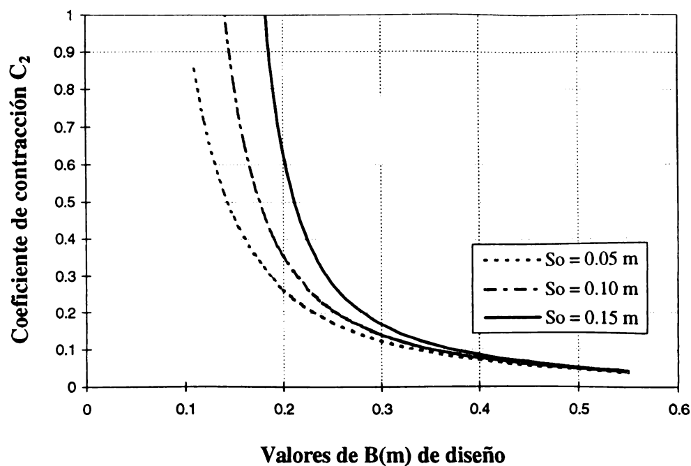
GRÁFICA 13. Ayuda de diseño, para rejillas con barras de \phi 5/8'' separadas 1.5 cm; para un caudal de 0.04 \text{ m}^3/\text{s/m} lineal de cresta de vertedero.
