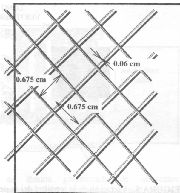
FIGURA 7b). Malla de “zaranda”.
