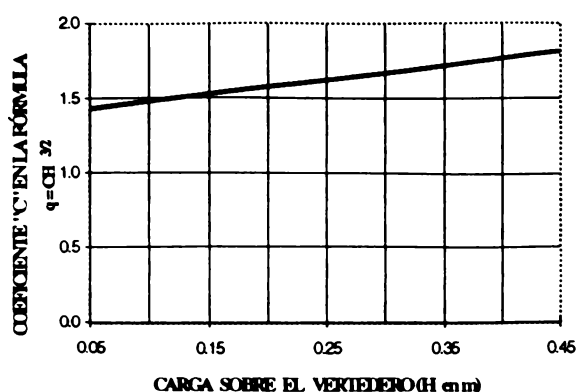
GRÁFICA 1. Coeficiente C en la fórmula general de vertederos rectangulares. Nyerges (2), p. 60.
