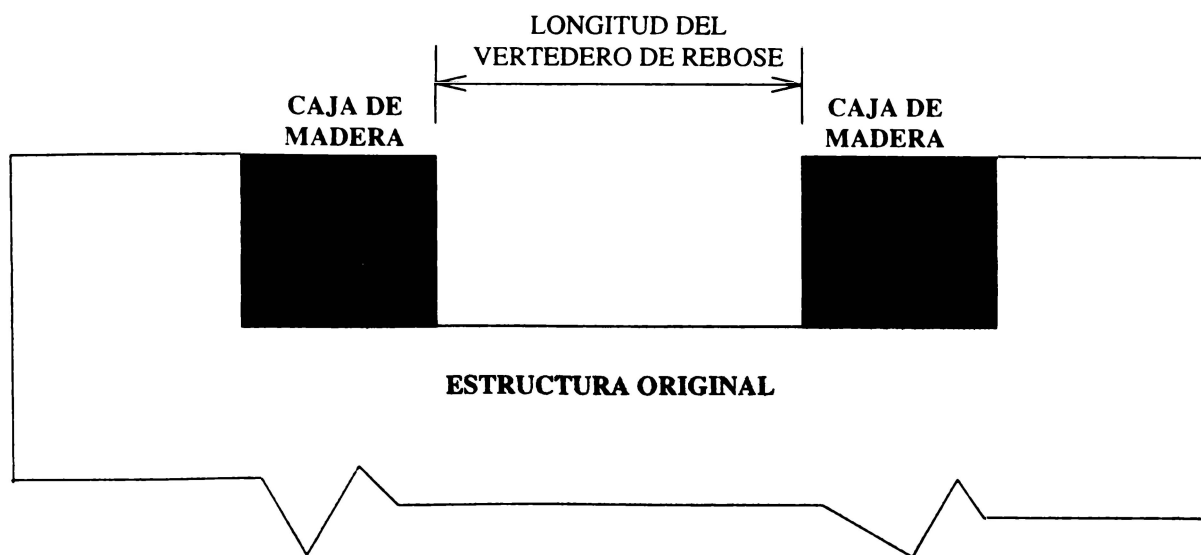
FIGURA 5. Variación de la longitud del vertedero de rebose por medio de cajas (vista frontal).
