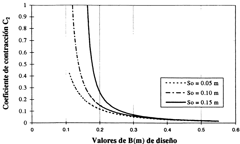
GRÁFICA 11. Ayuda de diseño para rejillas con barras de \phi 5/8'' separadas 1.5 cm; para un caudal de 0.02 \text{ m}^3/\text{s/m} lineal de cresta de vertedero.
