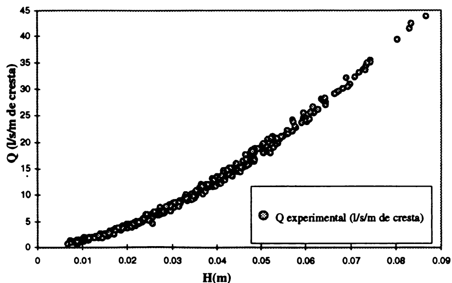
GRÁFICA 2. Valores medidos del caudal por metro lineal de cresta en función de H (m) experimental, para todos los casos.
