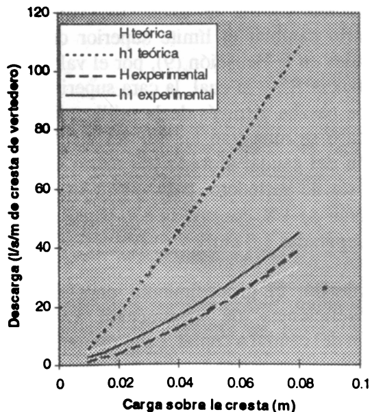
GRAFICA 7. Valores experimentales y teóricos de la descarga por metro lineal de cresta, en función de las cargas H y h_1 .
