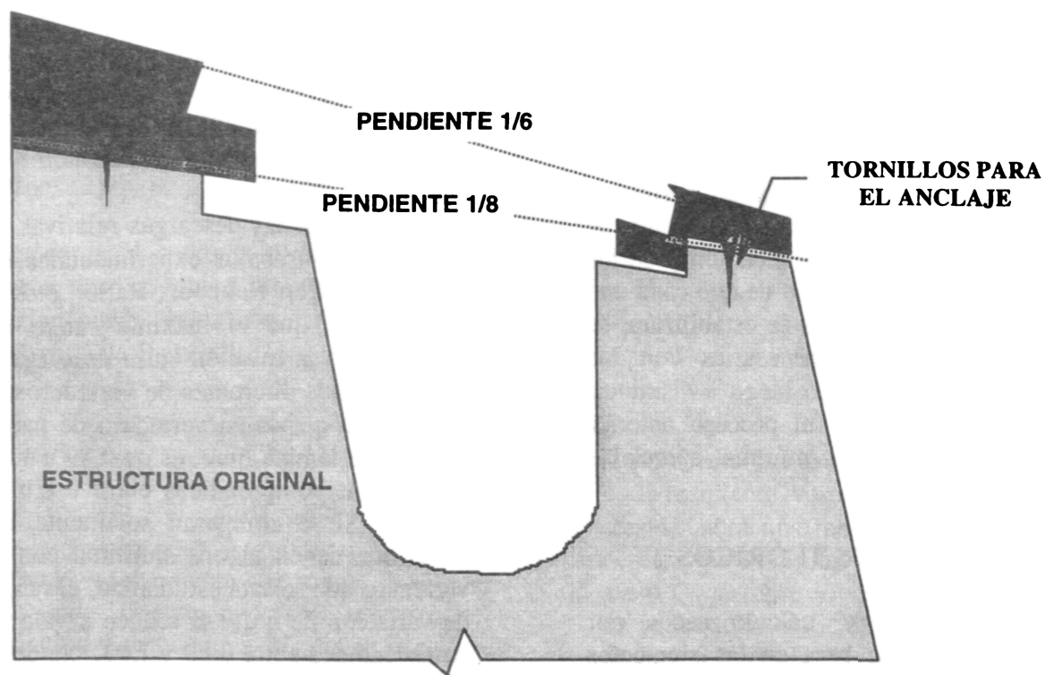
FIGURA 6. Variación de la pendiente de la cresta del vertedero (perfil).
