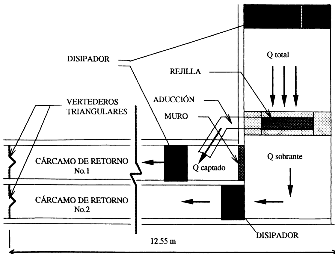
FIGURA 2. Esquema en planta del montaje realizado.
