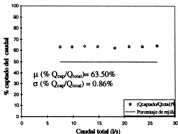
GRÁFICA 4. Porcentaje captado del caudal total, con rejilla de barras \phi 5/8'' separadas 1.5 cm ocupando un 50% del vertedero de rebose, con pendiente 1/8.
