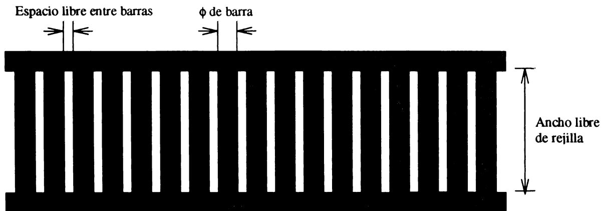
FIGURA 3. Variables de la rejilla involucradas en las expresiones teóricas.
