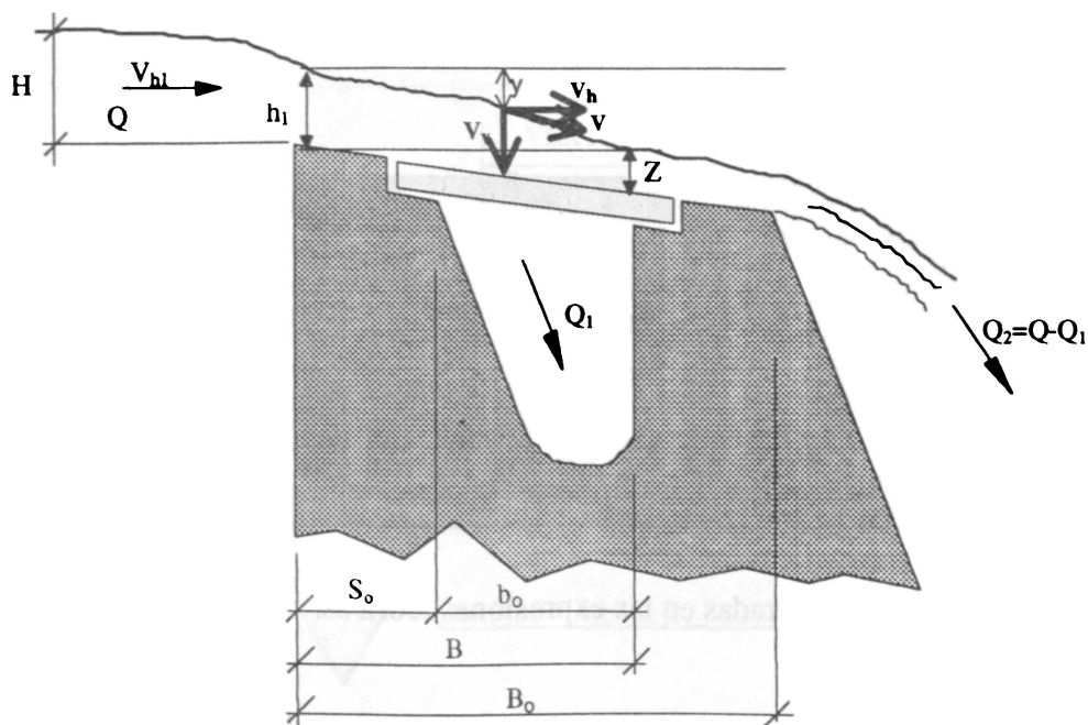
FIGURA 1. Variables de la estructura de captación involucradas en las expresiones teóricas. Nyerges (2), p. 56.
