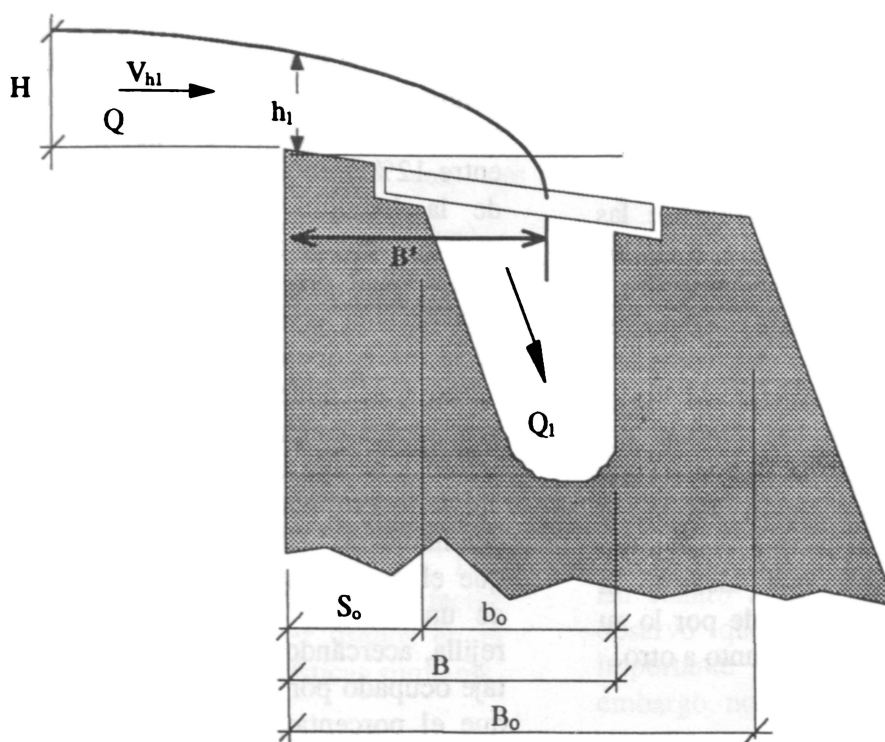
FIGURA 8. Distancia B' a la cual la cara superior de la napa entra a la rejilla.
