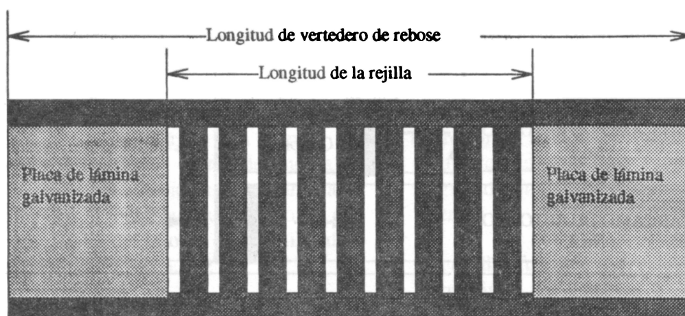
FIGURA 4. Variación de la longitud de la rejilla por medio de placa (vista en planta).
