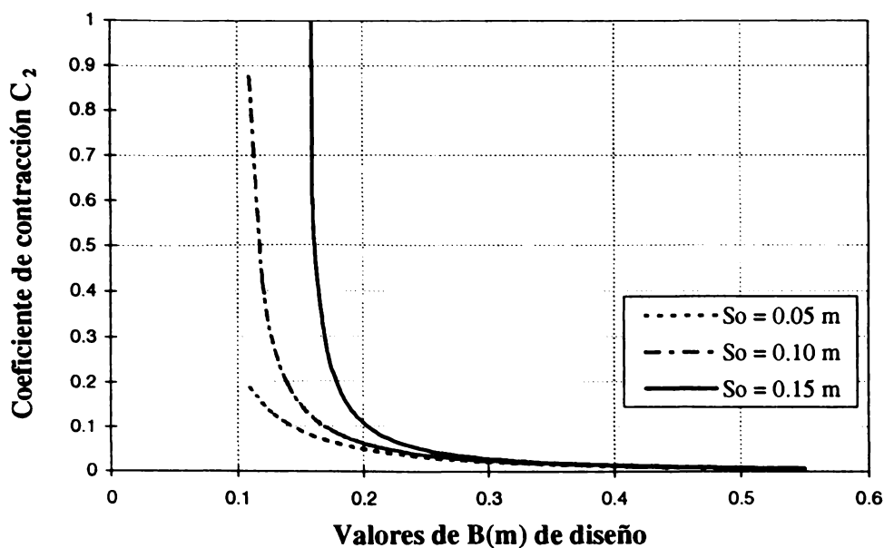
GRÁFICA 10. Ayuda de diseño para rejillas con barras de \phi 5/8'' separadas 1.5 cm; para un caudal de 0.01 \text{ m}^3/\text{s/m} lineal de cresta de vertedero.
