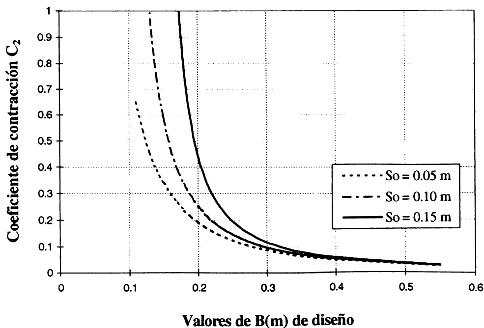
GRÁFICA 12. Ayuda de diseño para rejillas con barras de \phi 5/8'' separadas 1.5 cm; para un caudal de 0.03 \text{ m}^3/\text{s/m} lineal de cresta de vertedero.
