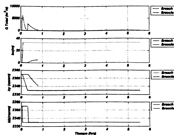
FIGURA 7. Comparación de resultados entre modelos Caso 4.
