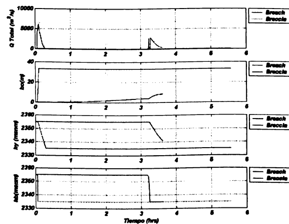
FIGURA 5. Comparación de resultados entre modelos, Caso 2
