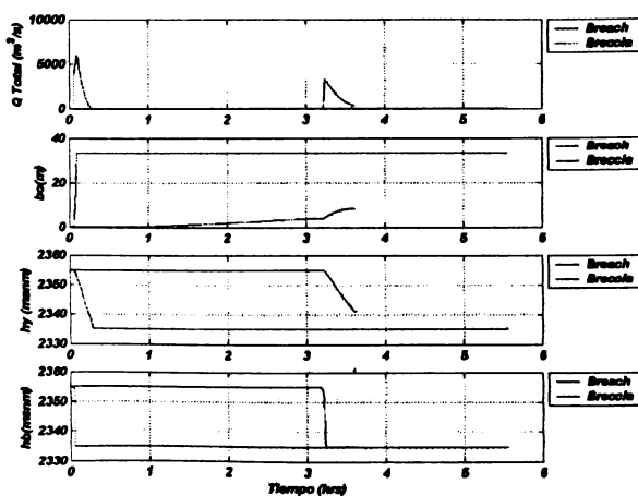
FIGURA 6. Comparación de resultados entre modelos, Caso 3
