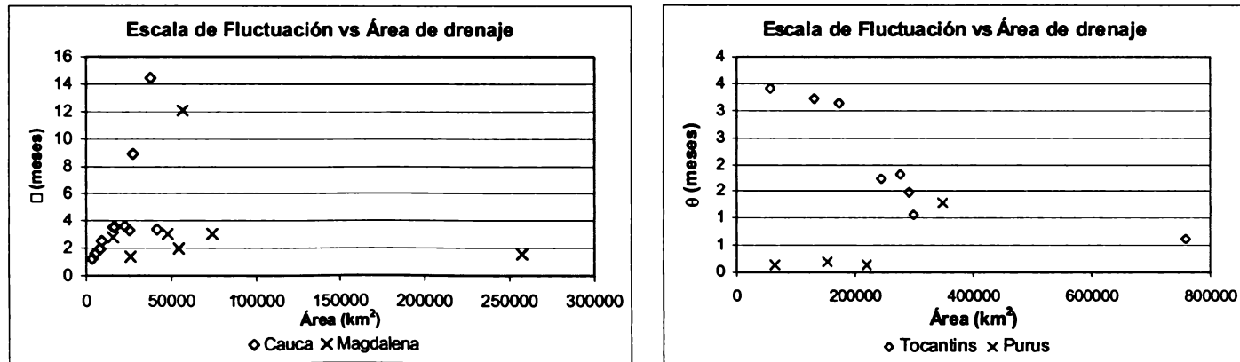
FIGURA 7. Relación entre la escala de Fluctuación estimada por el método del correlograma y el área de drenaje. Series de caudal en las cuencas de los Ríos Cauca y Magdalena (arriba) y en las cuencas de los Ríos Tocantins y Purus (abajo).
