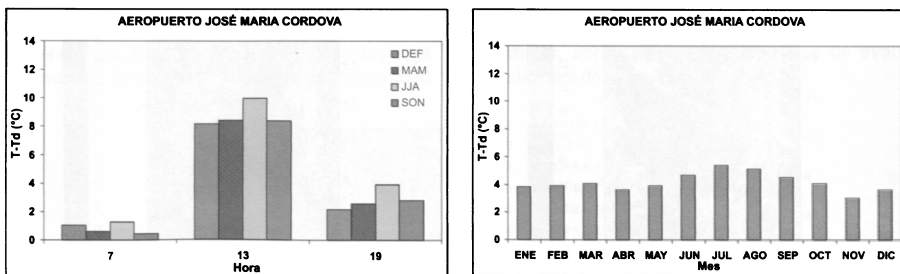
FIGURA 5. Gráficas de las diferencias entre la Temperatura media y Temperatura de Rocío para la estación del Aeropuerto José María Córdova, (a) Ciclo anual; (b) Ciclo diurno.
