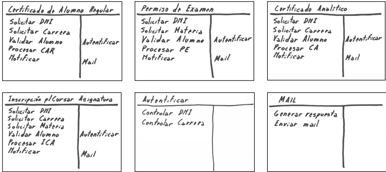
Figura 5. Tarjetas CRC del caso de estudio.
