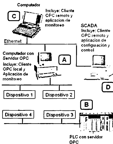
Figura 4: Planta industrial donde se ha implementado un sistema distribuido de monitoreo y control con OPC
