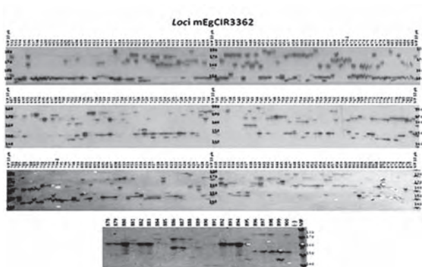
Figura 2. Patrón de amplificación del Locus mEgCIR3362. En cada columna se indica el patrón de amplificación de cada una de las 311 muestras de palma de aceite de Camerún. Donde MP representa el patrón de bandas del marcador de peso molecular y (-) es la columna correspondiente al control negativo.
