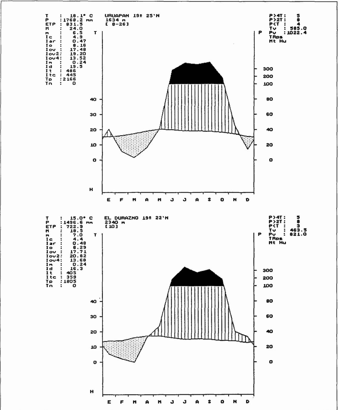
Figura 2. Diagramas bioclimáticos de las estaciones meteorológicas de Uruapan y El Durazno, elaborados con el programa Bioclima (Alcaraz 1995). En el extremo superior izquierdo se proporcionan los datos de temperatura media anual (T), precipitación medial anual (P), evapotranspiración (ETP), media de las máximas del mes más frío (M), media de las mínimas del mes más frío (m) y los diferentes índices bioclimáticos calculados.
