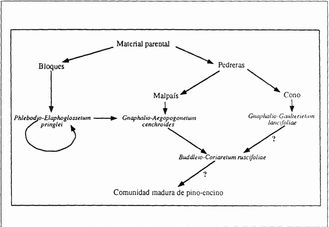
Figura 4. Modelo predictivo propuesto de la secuencia dinámica de las asociaciones vegetales del volcán Parícutín.
