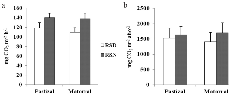
Figura 7. Tasas de respiración del suelo diurna y nocturna (RSD y RSN): a) medias mensuales (Anova, p > 0,05 , N = 60 ) y b) medias anuales en las dos fases sucesionales iniciales del bosque altoandino, cuenca del río Pamplonita.
