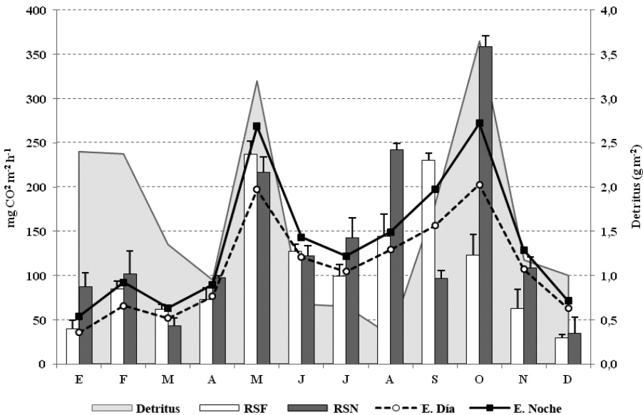
Figura 3. Comportamiento de la respiración del suelo diurna (RSD) y nocturna (RSN) en relación con la caída de detritus en el matorral de enero a diciembre de 2006. La línea continua indica la estimación de la respiración nocturna (E Noche) y la discontinua la diurna (E Día).
