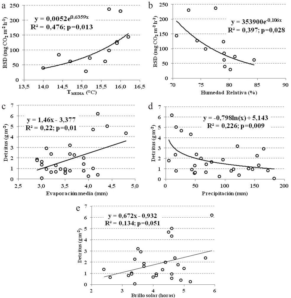
Figura 4. Relación de la respiración del suelo diurna (RSD) con: a) la temperatura media, b) la humedad relativa; y de la producción de detritus con: c) la evaporación, d) la precipitación y e) el brillo solar en el matorral de agosto de 2004 a diciembre de 2006.
