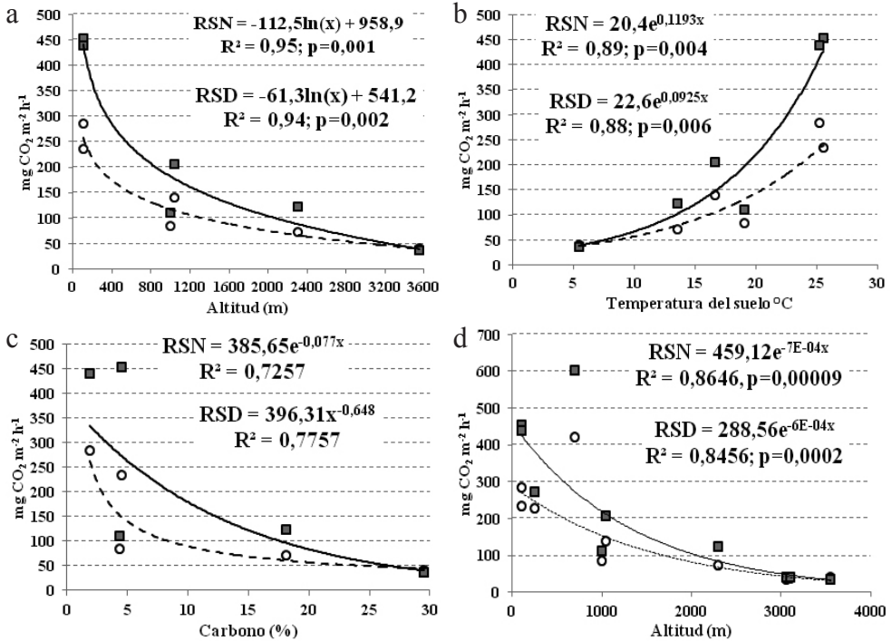
Figura 9. Relación de la respiración del suelo diurna RSD (círculo) y nocturna RSN (cuadrado) con: a) la altitud, b) la temperatura del suelo, el contenido de carbono y d) la altitud, en varias comunidades neotropicales de Venezuela y Colombia (Medina & Zelwer 1972, Cavelier & Peñuela 1990, Murcia & Ochoa 2008, Murcia 2010) modificado en este trabajo.
