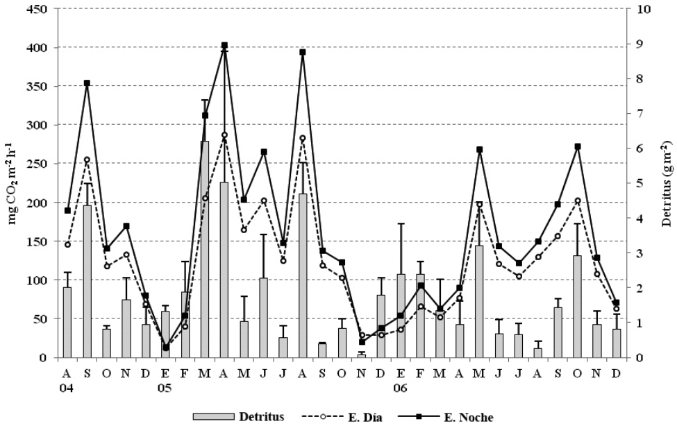
Figura 6. Comportamiento de la RSD y RSN estimadas con base en la dinámica de la temperatura media del aire y de la producción de detritus en el matorral de agosto de 2004 a diciembre de 2006.
