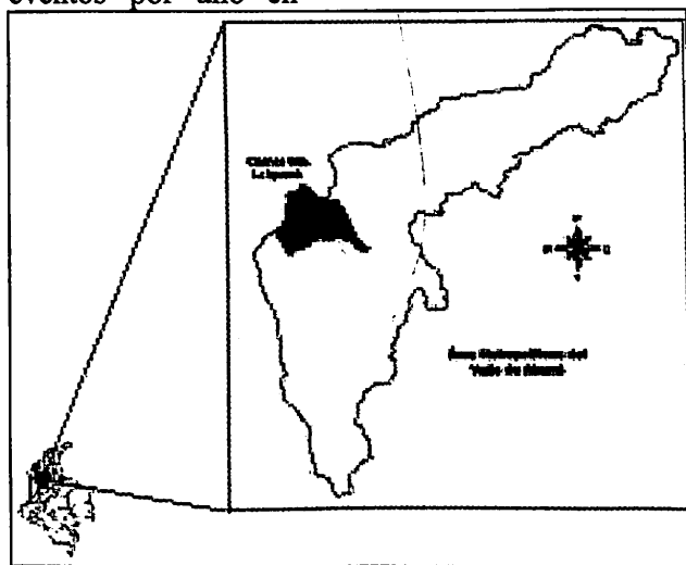
Figura 1. Ubicación de la zona de estudio
