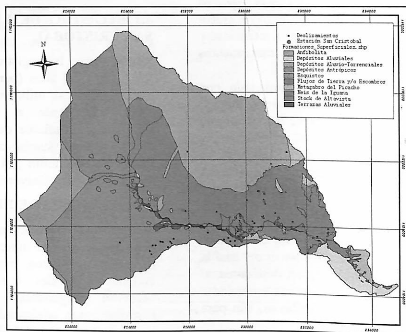
Figura 3. Mapa de formaciones superficiales (fuente Integral S.A.)
