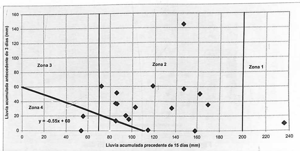
Figura 9. Deslizamientos y lluvia acumulada de 15 días.
