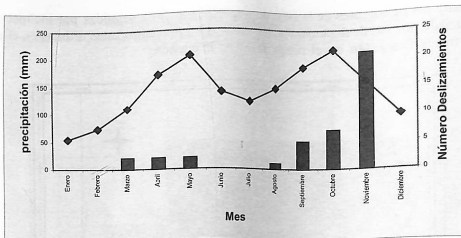
Figura 5. Relación precipitación promedio desde 1970-2001 y número de deslizamientos.
