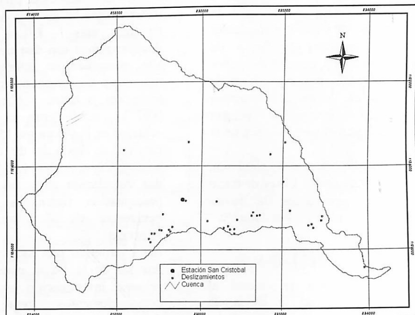
Figura 2. Ubicación de los deslizamientos en la zona de estudio.
