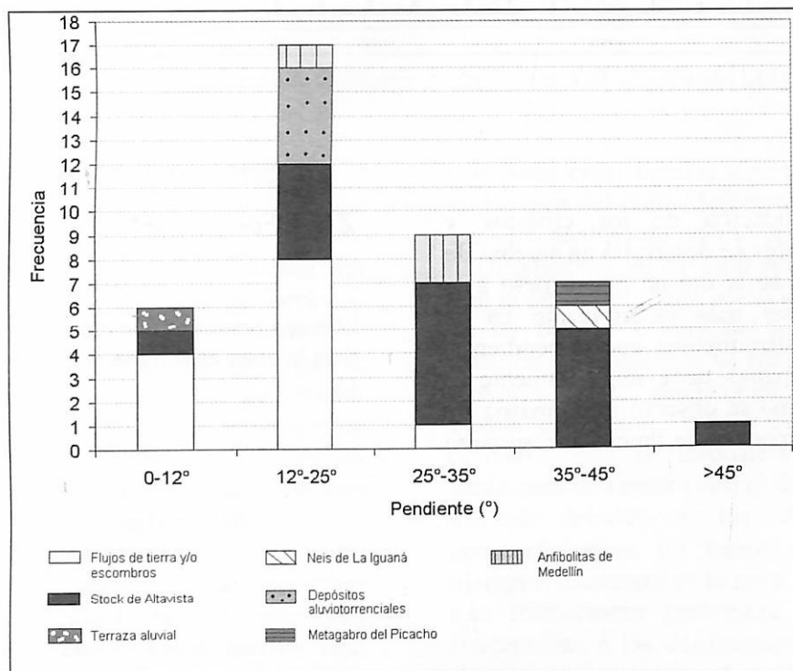
Figura 12. Pendiente del terreno y frecuencia de deslizamientos.
