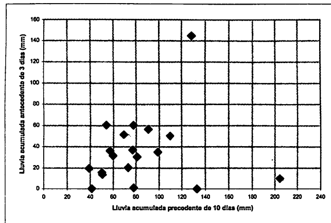
Figura 8. Lluvia acumulada de 10 días.
