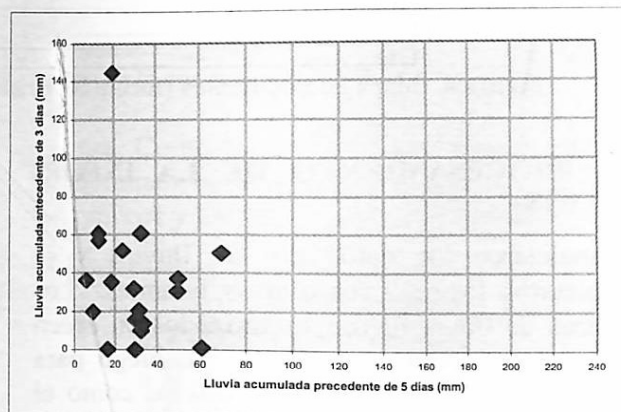
Figura 7. Lluvia acumulada de 5 días
