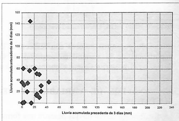
Figura 6. Lluvia acumulada de 3 días.
