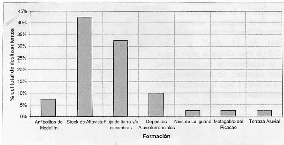
Figura 11. Formación superficial y deslizamientos.
