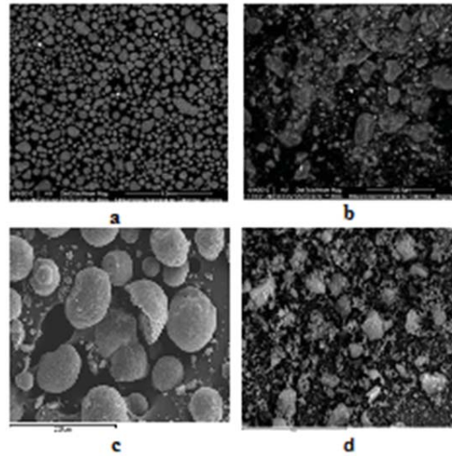
Figura 1. Imágenes por MEB de: a) FCC1 original, b) FCC1 molido, c) FCC2 original y d) FCC2 molido.
