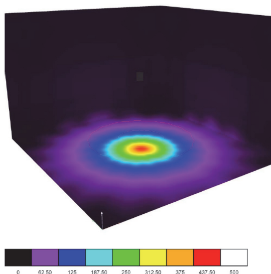
Figura 4: a) Izda. Gráfica de distribución lumínica (lux) de 200W LED mediante isolíneas en el plano del suelo (15x15m).
