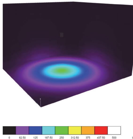
Figura 3: a) Izda. Gráfica de distribución luminica (lux) de 400W halogenuros metálicos mediante isocintas en el plano del suelo (15x15m).
