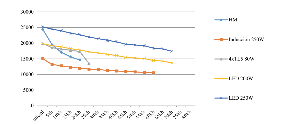
Figura 2. Gráfica comparativa de depreciación lumínica (lm) entre luminarias. Fuente: Elaboración propia.
