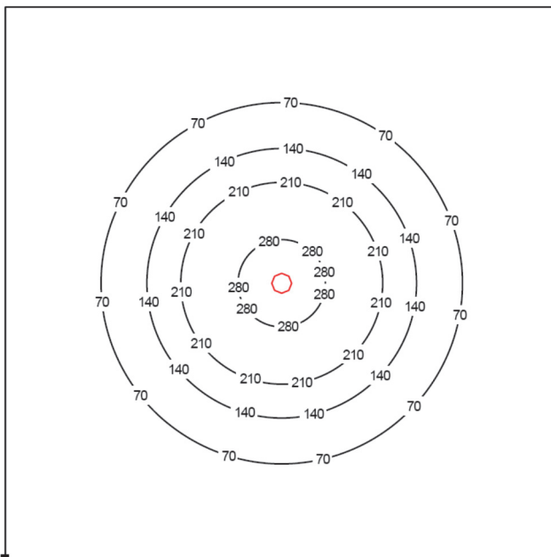
Figura 3: a) Izda. Gráfica de distribución luminica (lux) de 400W halogenuros metálicos mediante isocintas en el plano del suelo (15x15m).
