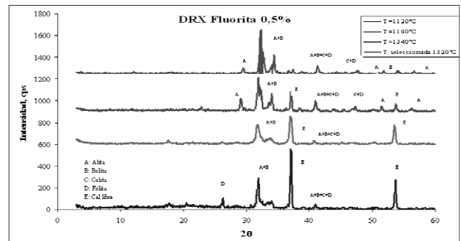
Figura 15. DRX Clínter con adición 0,5% de fluorita a diferentes temperaturas. Tiempo de residencia en el horno: 45min.
