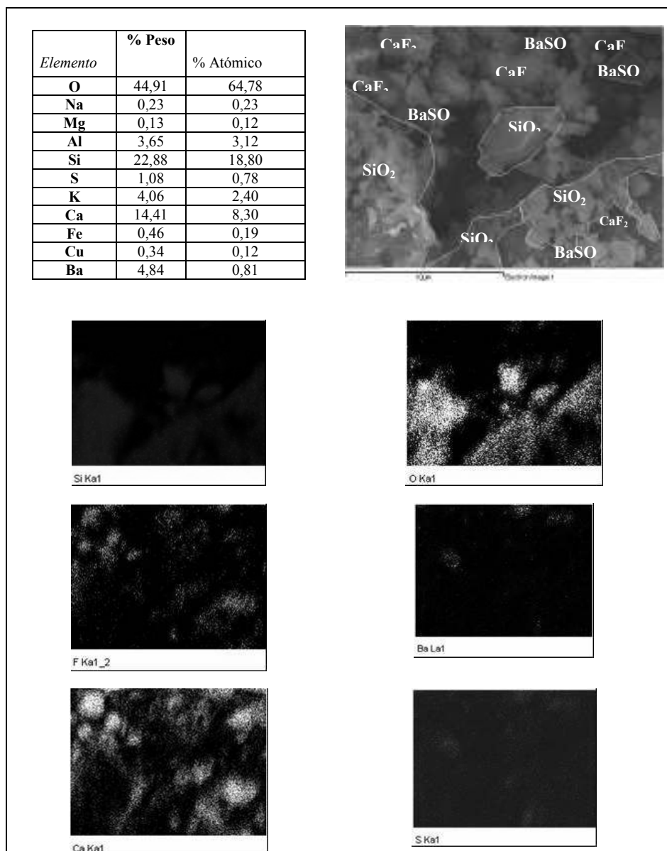
Figura 4. Caracterización de la Fluorita. SEM/WDS.
