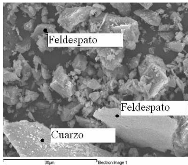
Figura 6. Caracterización del Feldespato. SEM/EDS. Figure 6. SEM/EDS of feldespar
