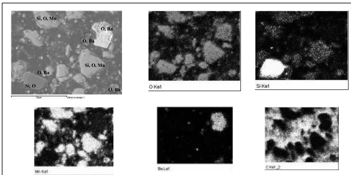
Figura 10. Caracterización del Manganeso. SEM/WDS.
