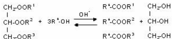
Figura 1. Representación general de la reacción de transesterificación entre una molécula de triglicérido y tres moléculas de alcohol.
