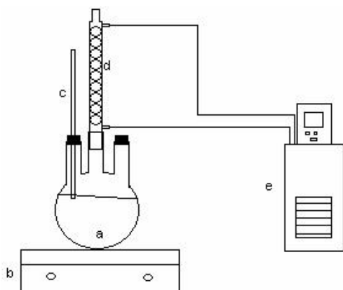
Figura 2. Montaje experimental para realizar la reacción de transesterificación: a. balón de tres bocas, b. manta de calentamiento con agitación magnética, c. termómetro de mercurio, d. condensador de reflujo, e. refrigerante.
