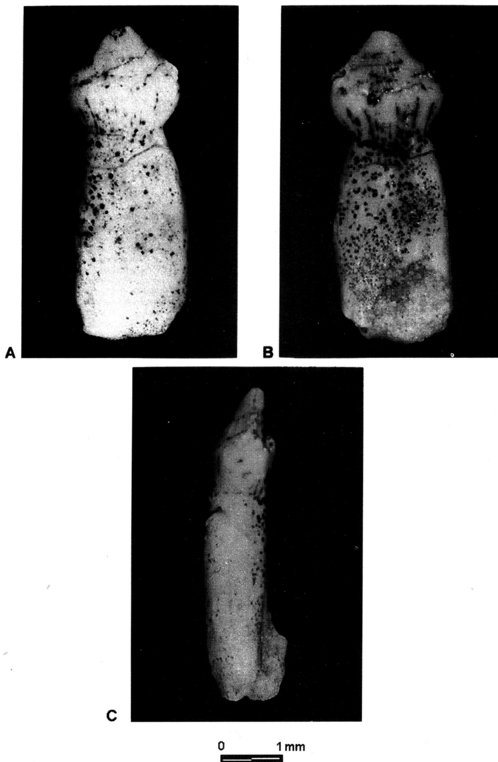
Fig. 10. Candidodon itapecuruense (MN-4154-V) Dente molariforme. Holótipo. (A) face bucal; (B) face lingual; (C) vista lateral.
