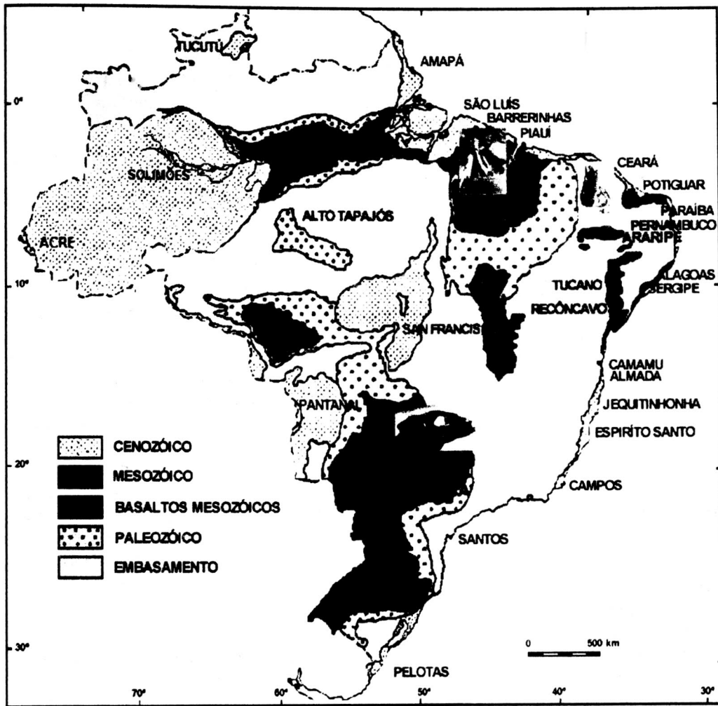
Fig. 1. Distribuição das principais bacias cretácicas brasileiras e indicações das ocorrências de nostossúquios.
