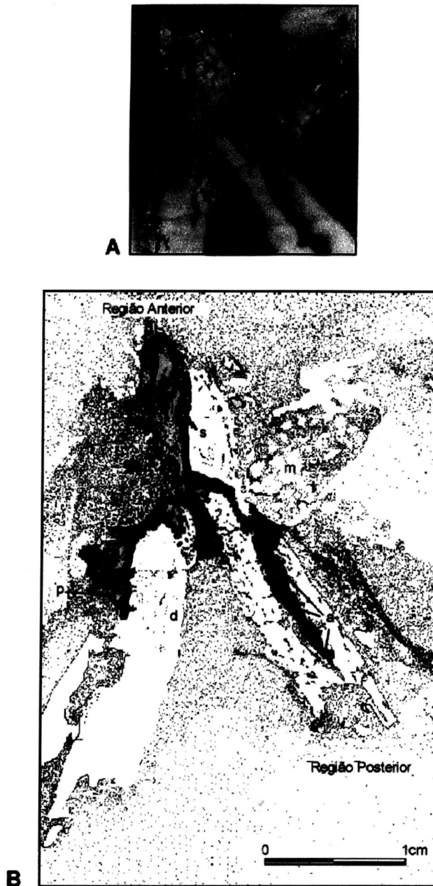
Fig. 12. Candidodon itapecuruense (MN-4355-V), espécimen na Formação Itapecuru, Bacia do Parnaíba. Mandíbula com os dois ramos mandibulares. (A) Fotografia em vista dorsal; (B) Desenho esquemático da mandíbula.
