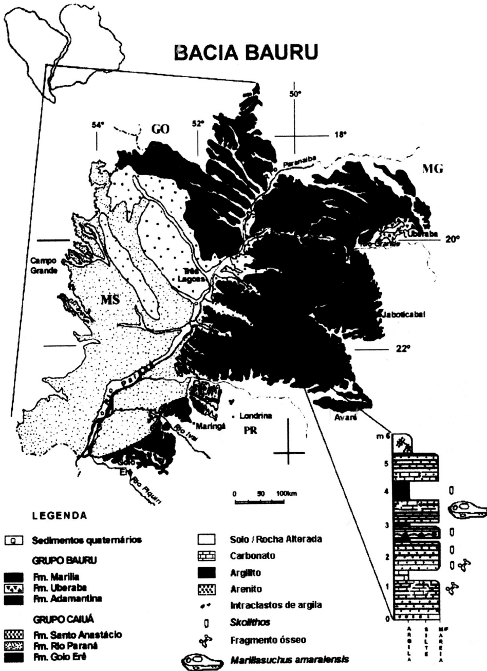
Fig. 15. Mapa geológico da Bacia Bauru, e perfil estratigráfico da região ao sul de Marília, de onde é proveniente Mariliasuchus amarali . Modificado de FERNANDES & COIMBRA (1996).
