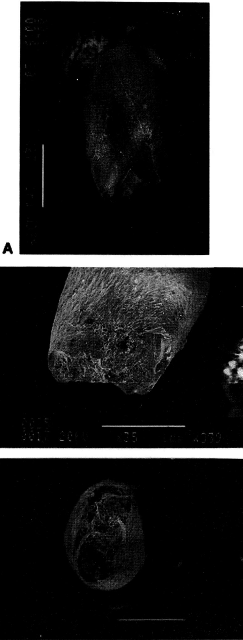
Fig. 13. Candidodon itapecuruense (MN-4356-V). Fotomicrografias de um dente molariforme. (A) Superfície lingual do dente; a região próxima à raiz apresenta-se deprimida, formando um sulco amplo na base da raiz uniradiculada; (B) detalhe da base da raiz; (C) aspecto bifurcado da base da raiz.
