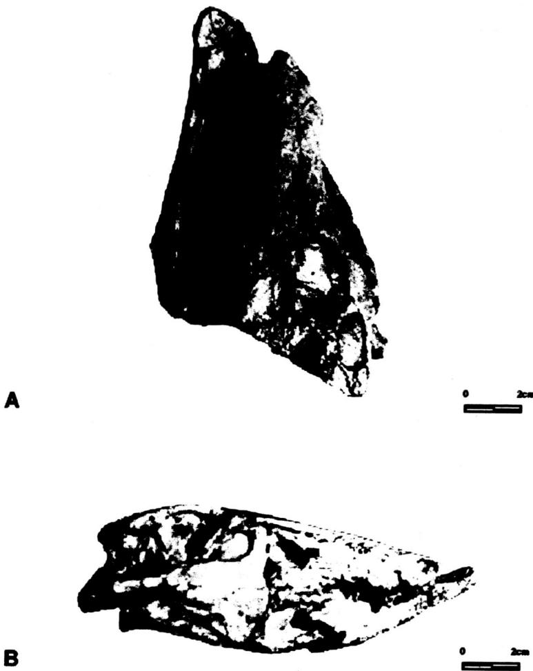
Fig. 5. Araripesuchus gomesii (Holótipo: DGM 423 - R) oriundo da localidade de Ladeira do Berlenga, Piauí. Bacia do Araripe, Formação Santana (Aptiano-Albiano).
