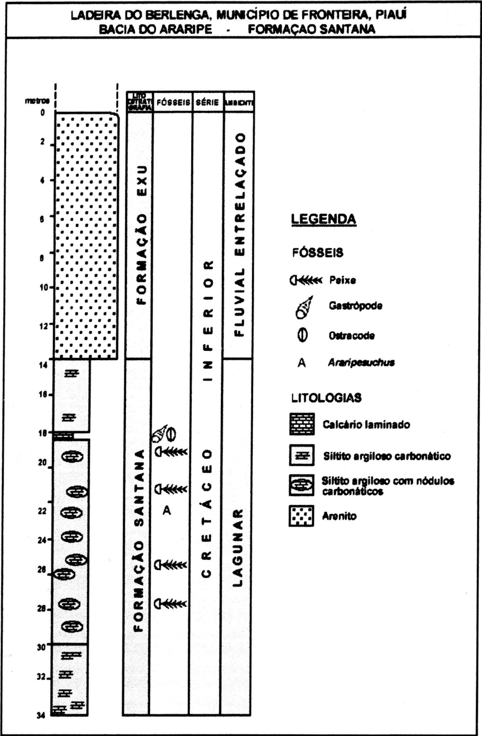
Fig. 4. Perfil estratigráfico da Ladeira do Berenga, Estado do Piauí, localidade de onde provém Araripesuchus .
