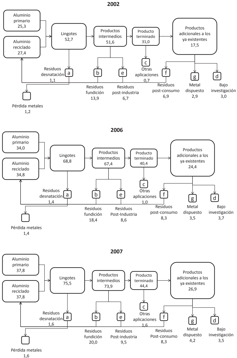
Figura 2. Flujo mundial del aluminio 2002, 2006 y 2007. a) aluminio desnataado; b) residuos de fundición, rollos y extrusión; c) aplicaciones del aluminio (de-ox, polvo); d) investigación sobre destino final del aluminio (recuperación, reciclaje o disposición); e) residuos de producto terminado; f) residuos consumo masivo; g) material dispuesto. Fuente: elaboración propia a partir de European Aluminum Association (2004), The Global Aluminum Recycling Committee (2006), Kamberović et al. (2009), Menzie et al. (2010), Dahmus (2014).
