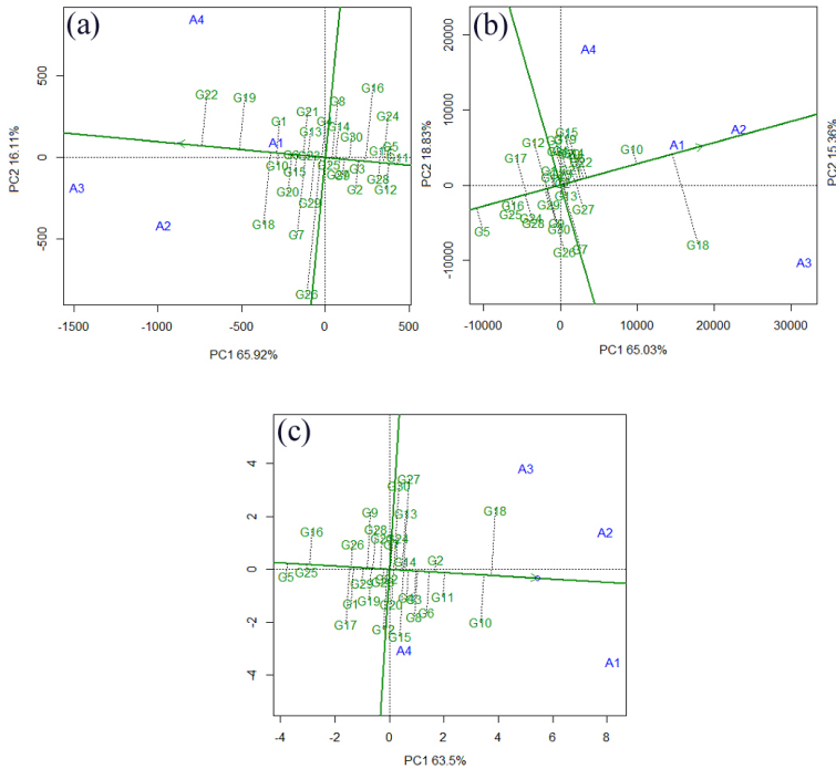
Figura 2. O GGE biplot (“Média versus Estabilidade”) com eixo do ambiente-média (EAM) para mostrar o desempenho médio e estabilidade dos genótipos para as características peso médio dos cachos (a), peso total de cachos (b) e número total de cachos (c) em progênies de açaizeiro, quais dos genótipos apresentaram melhor desempenho em que ambientes.
