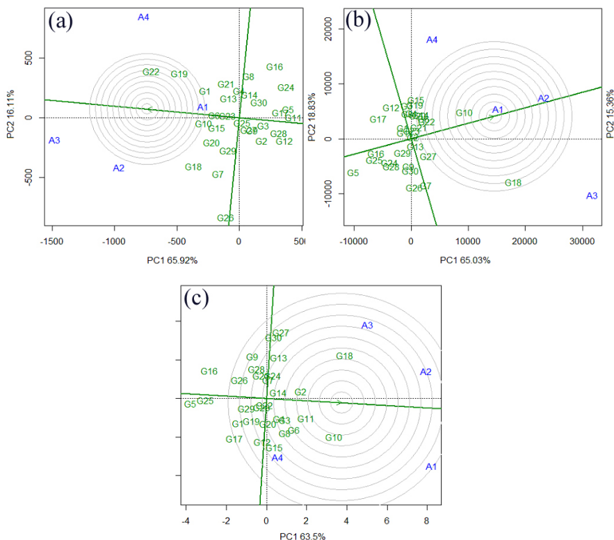
Figura 3. O GGE biplot com eixo do ambiente-média (EAM) para classificar os genótipos em relação ao ideótipo (no centro dos círculos concêntricos) para as características peso médio dos cachos (a), peso total de cachos (b) e número total de cachos (c) em progênies de açaizeiro, quais dos genótipos apresentaram melhor desempenho em que ambientes.
