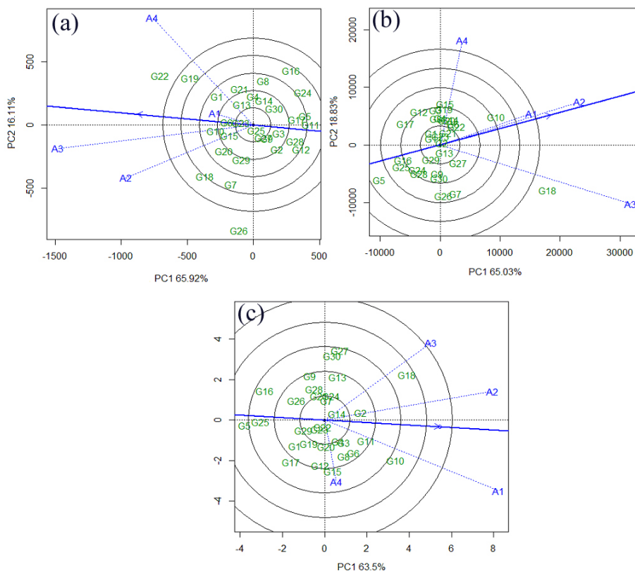
Figura 4. O GGE biplot “discriminação e representatividade” para mostrar a capacidade de discriminação e representatividade dos ambientes de teste nas características peso médio dos cachos (a), peso total de cachos (b) e número total de cachos (c) em progênies de açaizeiro, quais dos genótipos apresentaram melhor desempenho em que ambientes. Anajás, PA.
