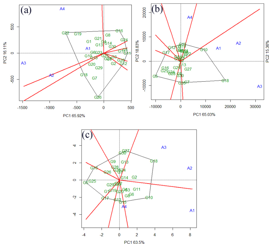
Figura 1. O GGE biplot (“Which-won-where”) para os dados das características peso médio dos cachos (a), peso total de cachos (b) e número total de cachos (c) em progênies de açaizeiro, quais dos genótipos apresentaram melhor desempenho em que ambientes.
