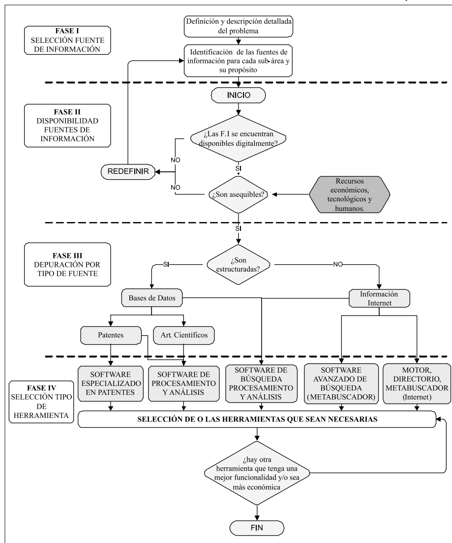
Figura 2. Metodología para la selección de herramientas de software para la VT
