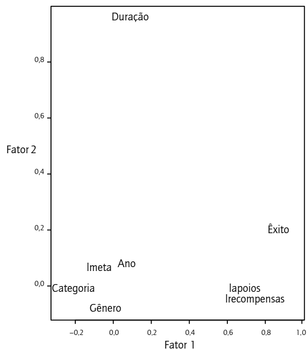
Figura 2. Agrupamento das variáveis em função das correlações existentes Nota: essa figura apresenta o agrupamento das variáveis de interesse em função dos níveis de correlações existentes. Fonte: elaboração própria.
