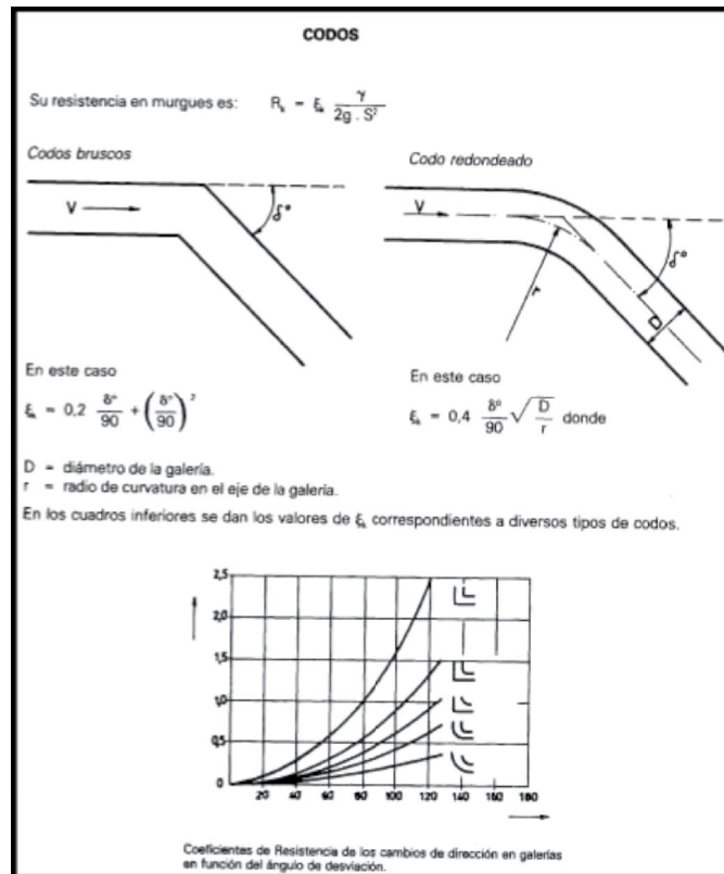
Figura 1. Cálculo de la resistencia asociada a un codo. Fuente: Leal (2003).
