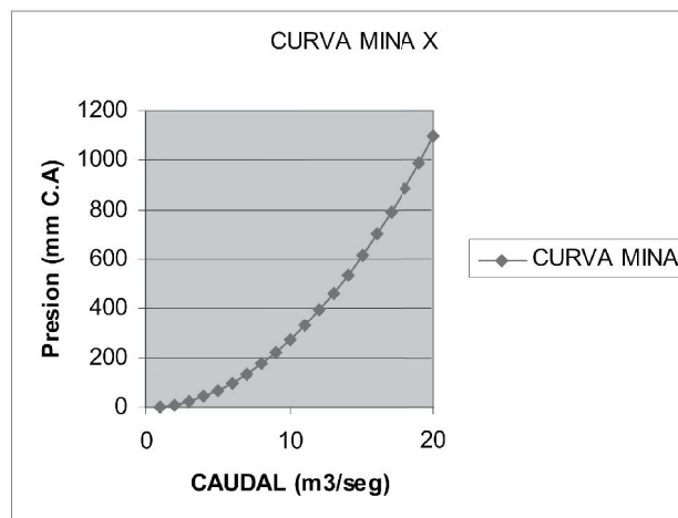
Figura 2. Curva característica de una mina (Datos de Ejemplo)
