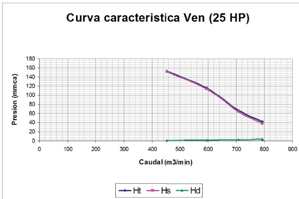
Figura 4. Curva característica de una mina.
