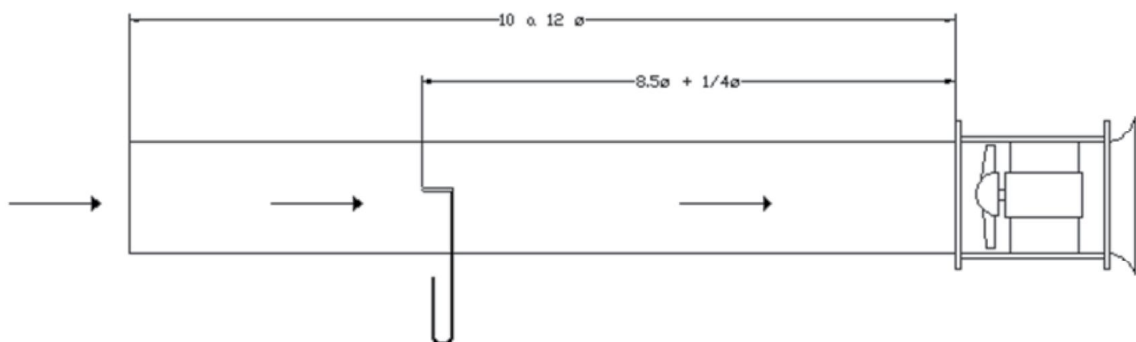
Figura 3. Túnel de viento .Fuente: Gómez G. (2007).
