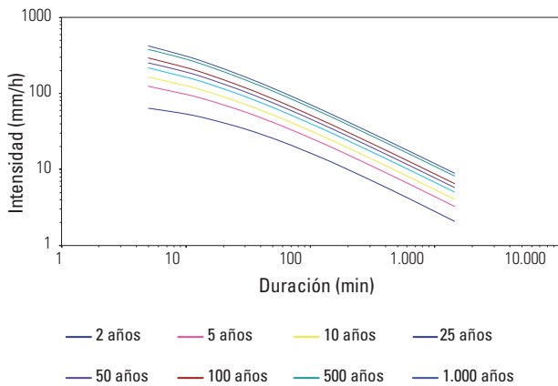
Figura 10. Curvas de profundidad-duración-frecuencia (PDF) ajustadas por el método de Wenzel para láminas máximas anuales de precipitación (periodo 1974-1999) de la estación Macuto, estado Vargas, Venezuela. Datos: elaborado a partir de las láminas máximas anuales de precipitación de la estación Macuto del Instituto Nacional de Meteorología e Hidrología (2013b), ajustadas por el método de Wenzel (1982).
