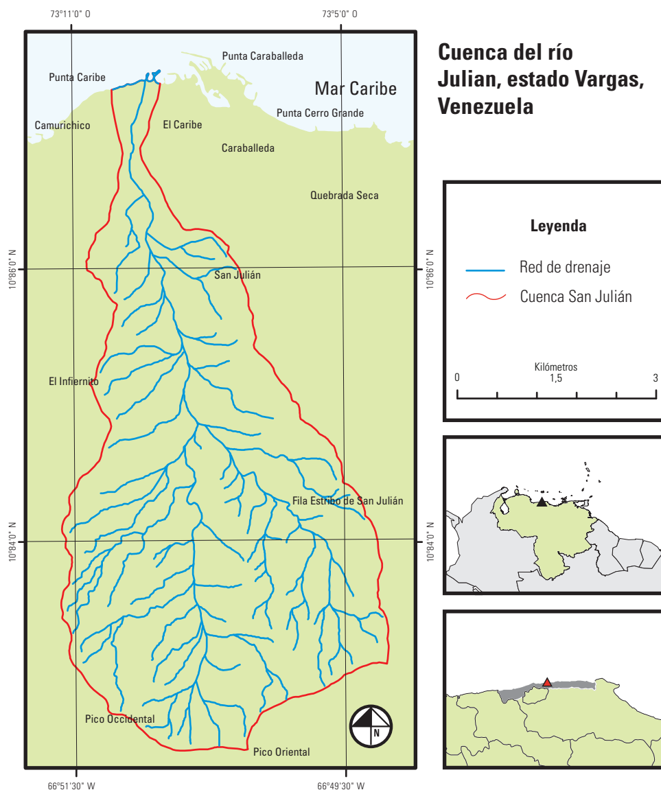
Figura 5. Red de drenaje del río San Julián, estado Vargas, Venezuela. Datos: base cartográfica de la Dirección de Cartografía Nacional (1979).
