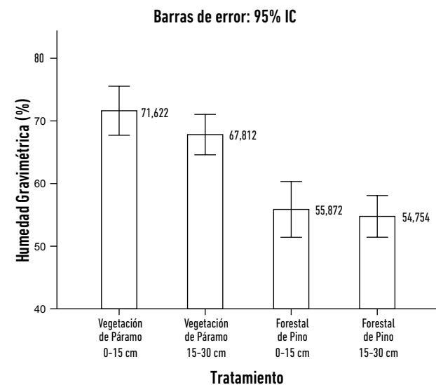
Figura 10. Humedad gravimétrica del suelo en los diferentes tratamientos.
