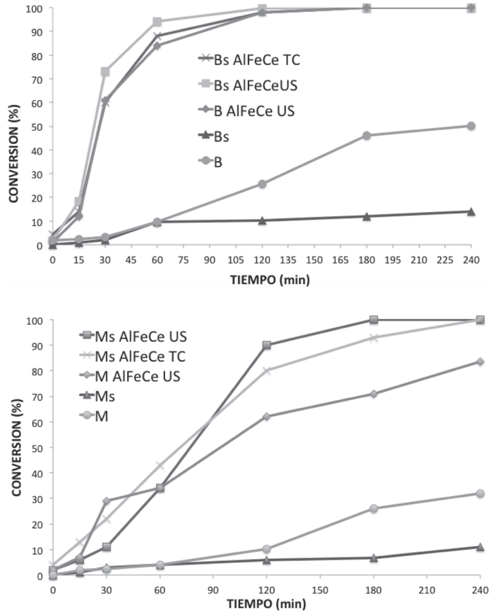
Figura 6. Conversión de fenol en función del tiempo de reacción para los sólidos con previa remoción de hierro
