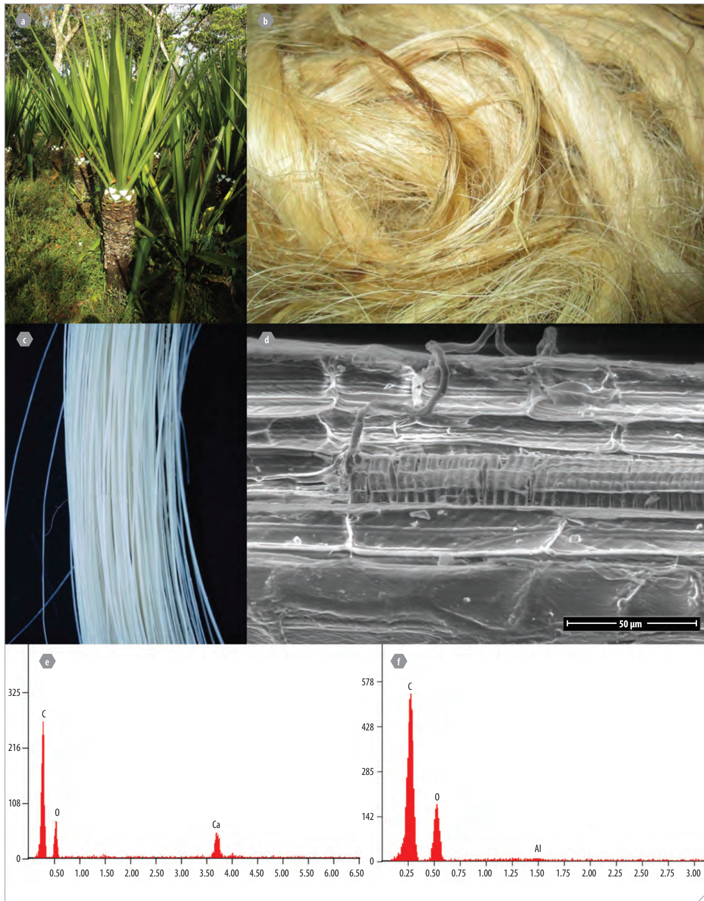
Figura 1. a. Planta de fique. b. Fibras de fique sin tratamiento. c. Fibras de fique limpias. d. Micrografía de una fibra de fique (magnificación de 1500X). e. Espectro EDX de fibras de fique crudas. f. Espectro EDX de fibras de fique limpias.
