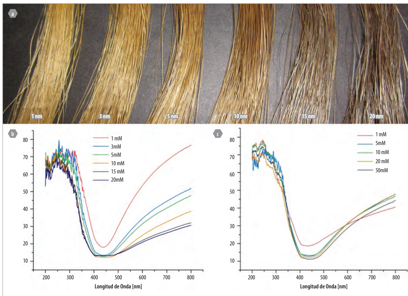
Figura 3. a. Apariencia de las fibras de fique modificadas con Ag NPs cuando varía la concentración de AgNO 3 . b. Espectros de reflectancia difusa que se obtienen bajo diferentes concentraciones de AgNO 3 . c. Espectros de reflectancia difusa que se logran al modificar la concentración de NaBH 4 .
