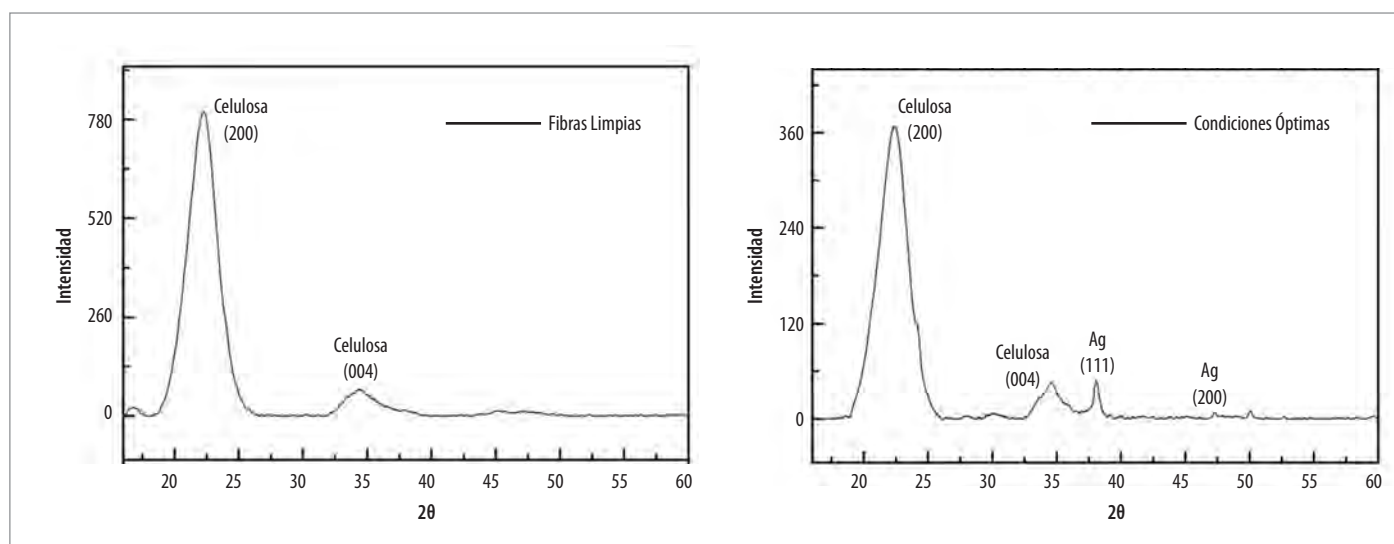
Figura 5. Difractogramas de las fibras de fique limpias y de los bionanocompositos de fibras de fique y nanopartículas de plata sintetizados bajo condiciones óptimas.
