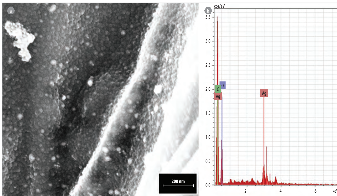
Figura 4. a. Micrografía SEM de las fibras modificadas con Ag NPs bajo condiciones óptimas de síntesis (magnificación de 300000X). b. Espectro EDX de las fibras modificadas con Ag NPs utilizando condiciones óptimas de síntesis.
