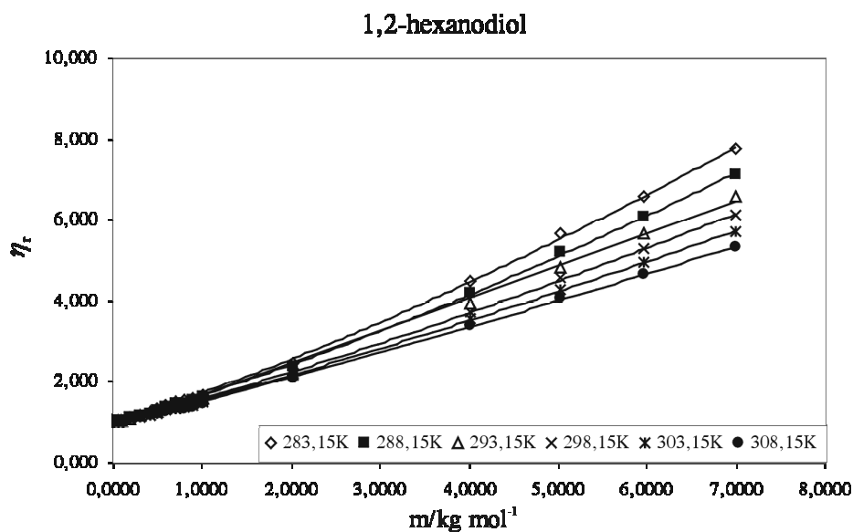
Figura 1. Viscosidad relativa de soluciones acuosas diluidas de 1,2-hexanodiol a 283,15; 288,15; 293,15; 298,15; 303,15 y 308,15 K.
